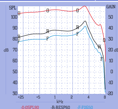
EN 60118-7:2005 2ccm-coupler
